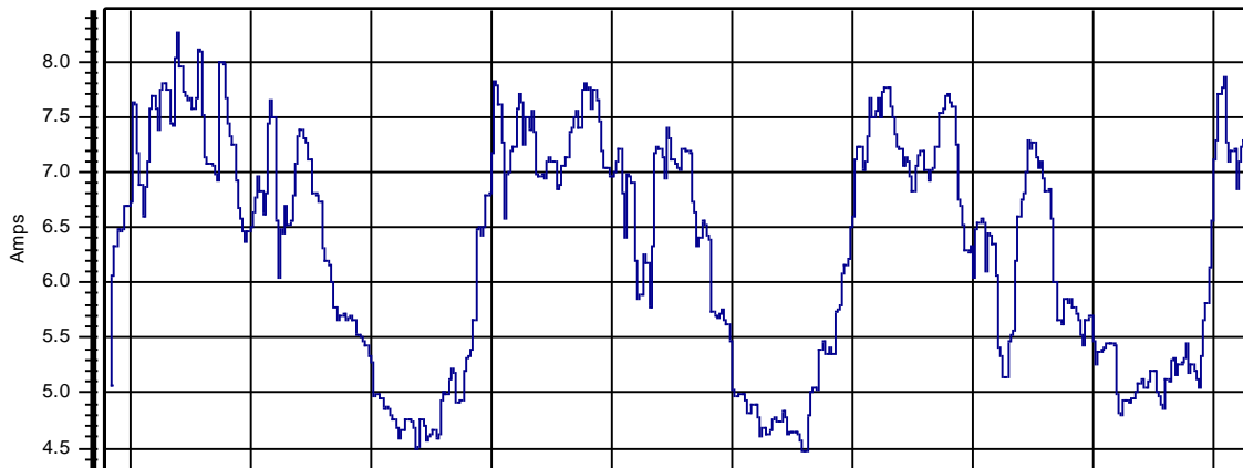
— C IHam(450Hz)
