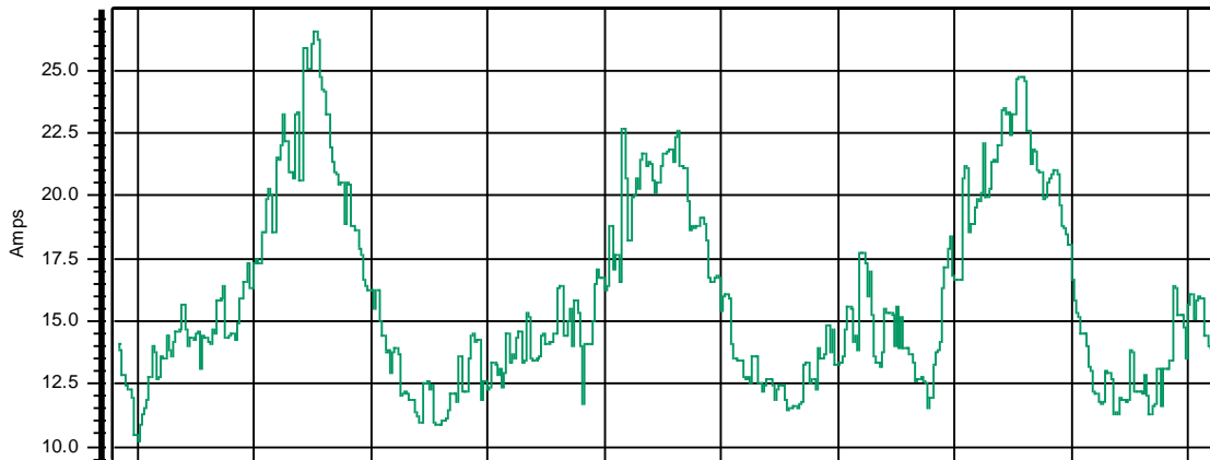
— B IHam(150Hz)
