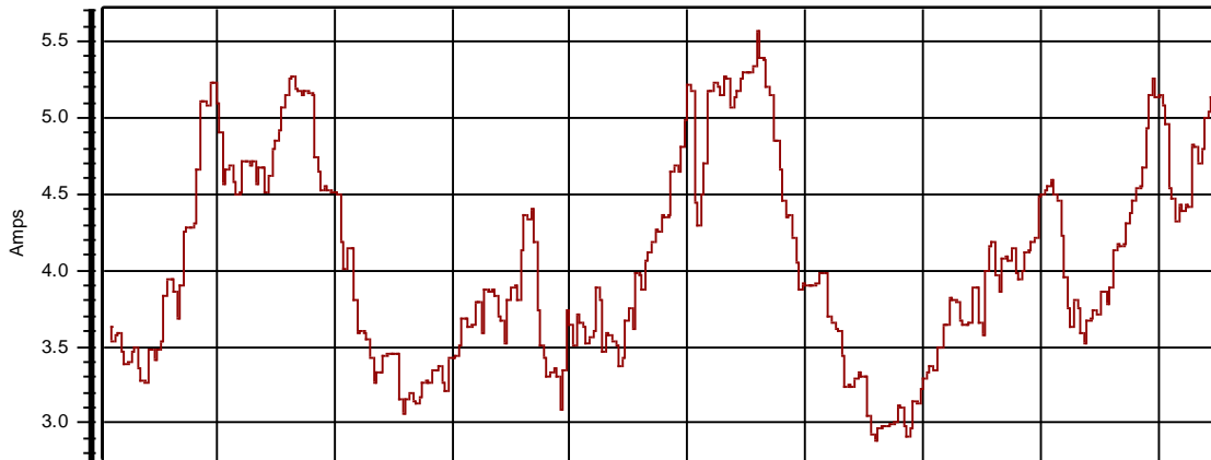
— A IHam(450Hz)
